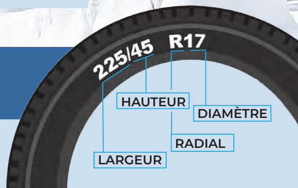
LIRE LA DIMENSION D'UN PNEU
